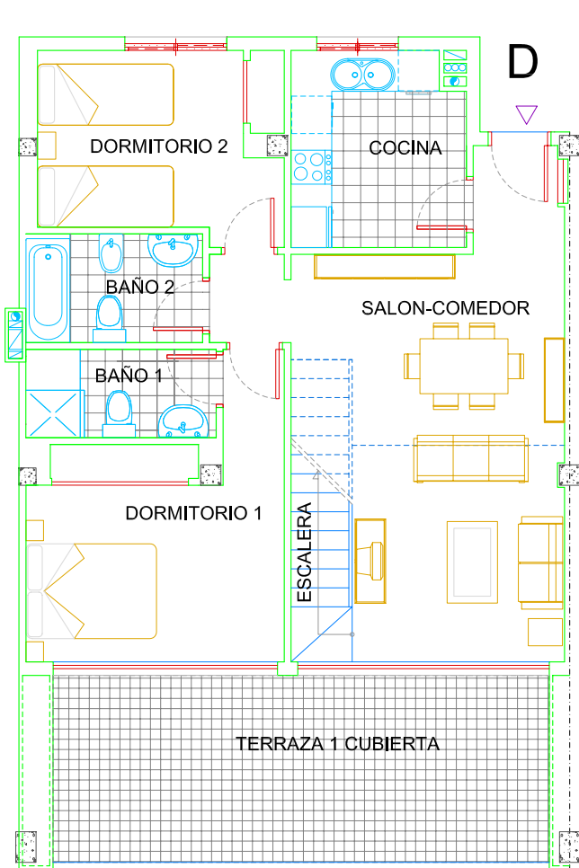
PLANTA SEGUNDA
